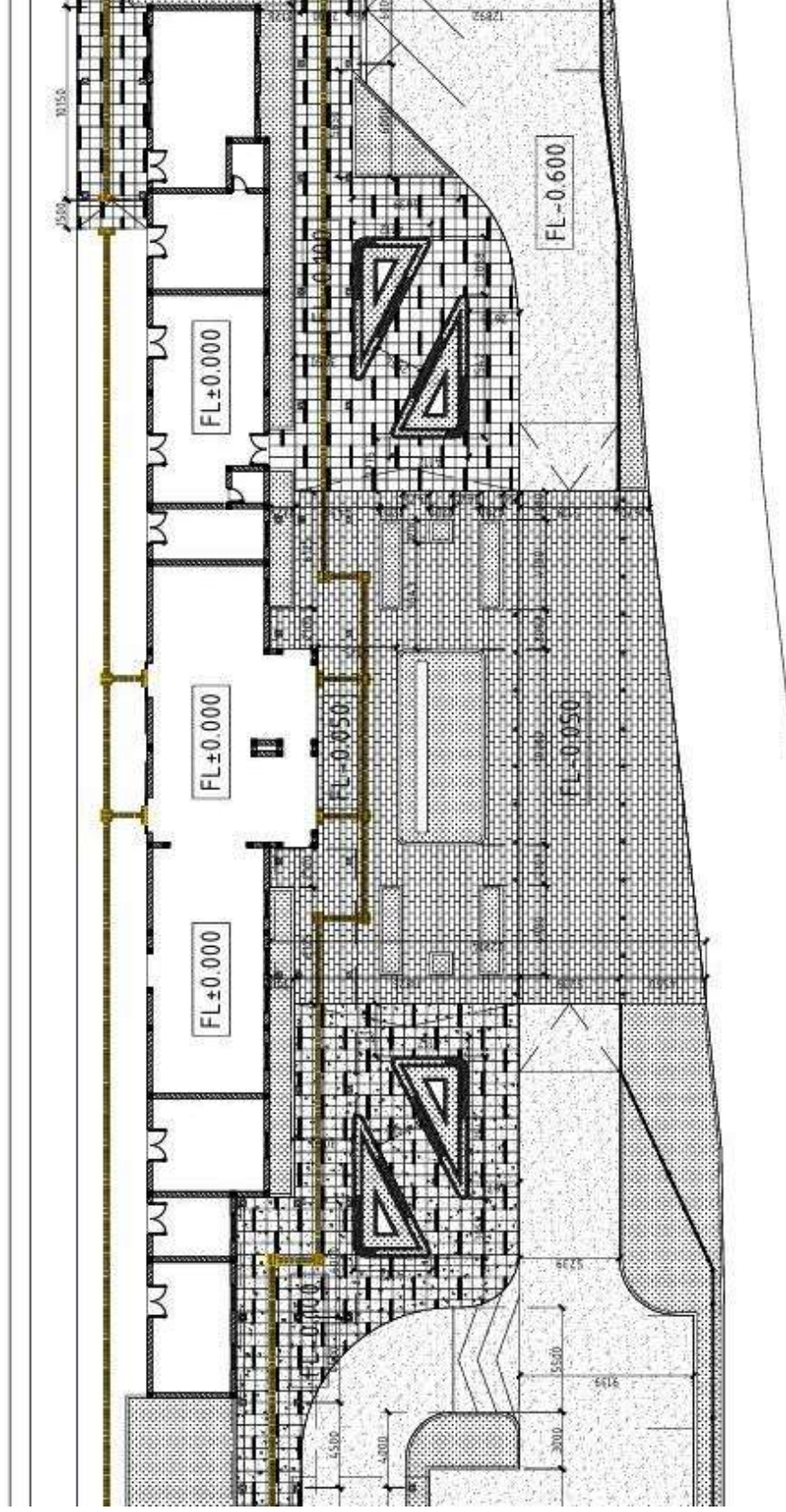
Lampiran 2. Site Plan Bangunan Utama
