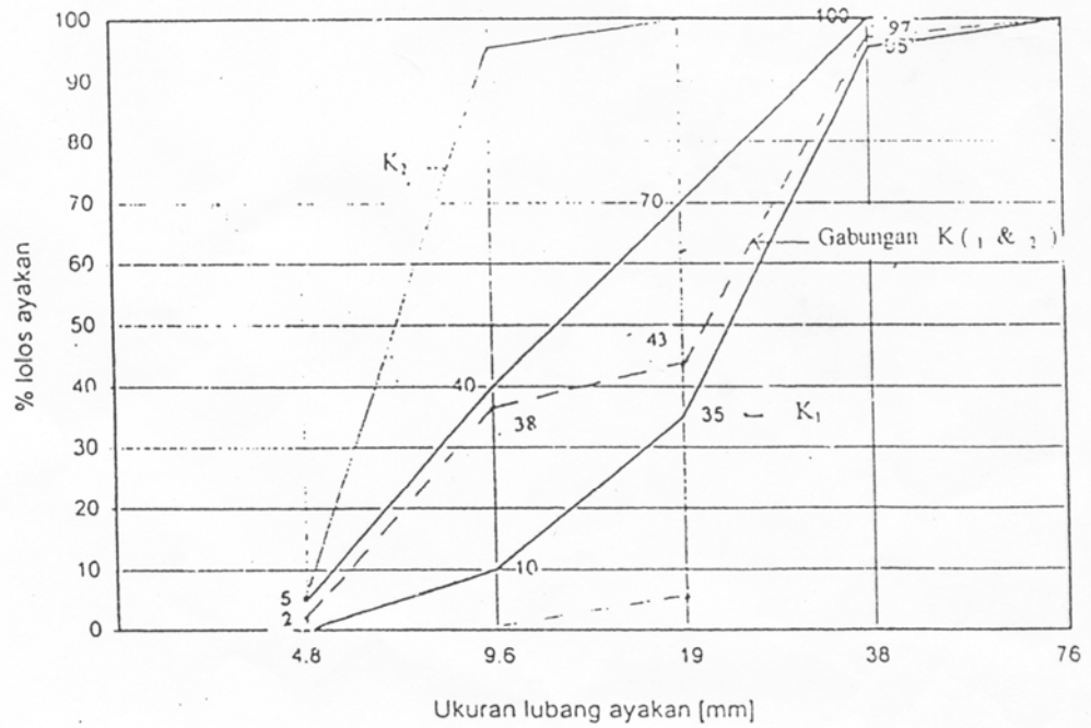
Grafik 19 Batas Gradasi atau Korat Ukuran Maksimum 40 Mm
