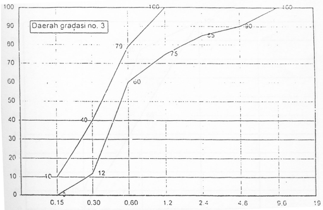
Grafik 4 Batas Gradasi Pasir (Sedang) No. 2
