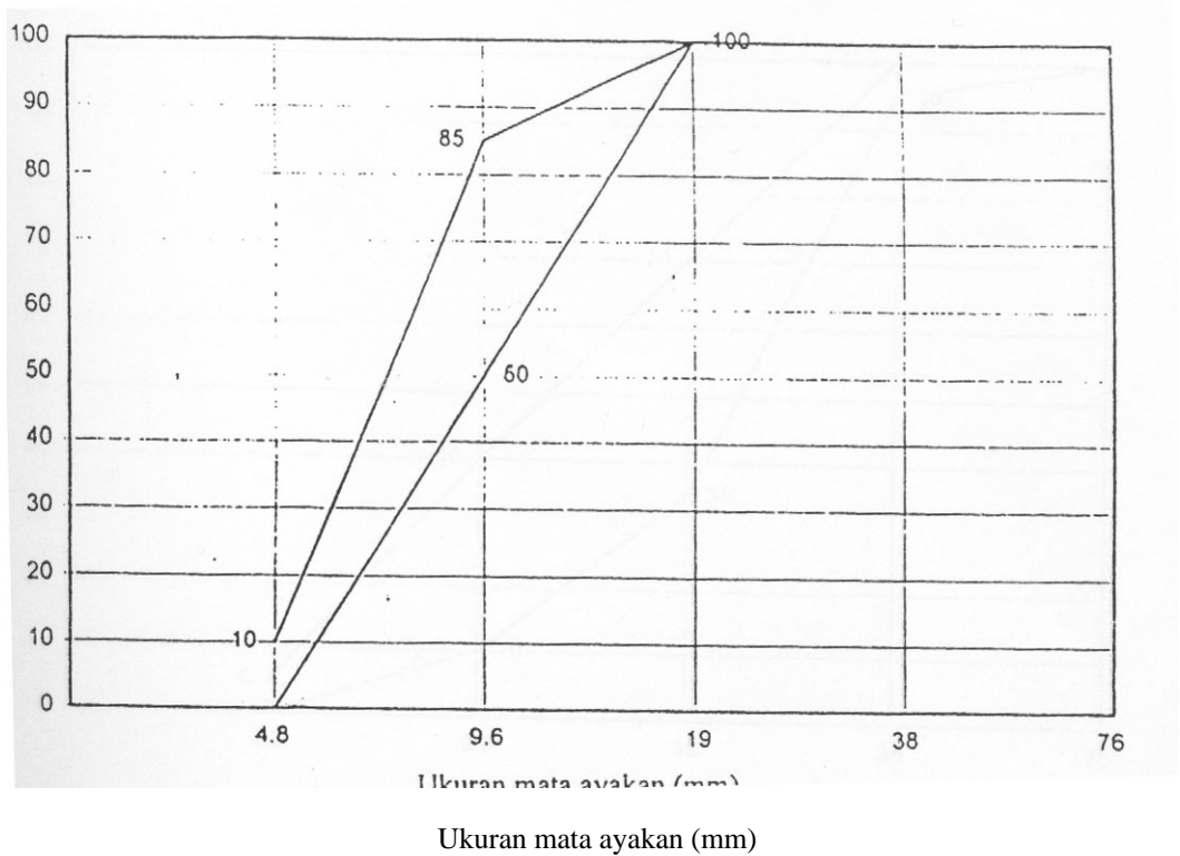
Grafik 7 Batas gradasi kerikil atau koral ukuran maksimum 10 mm
