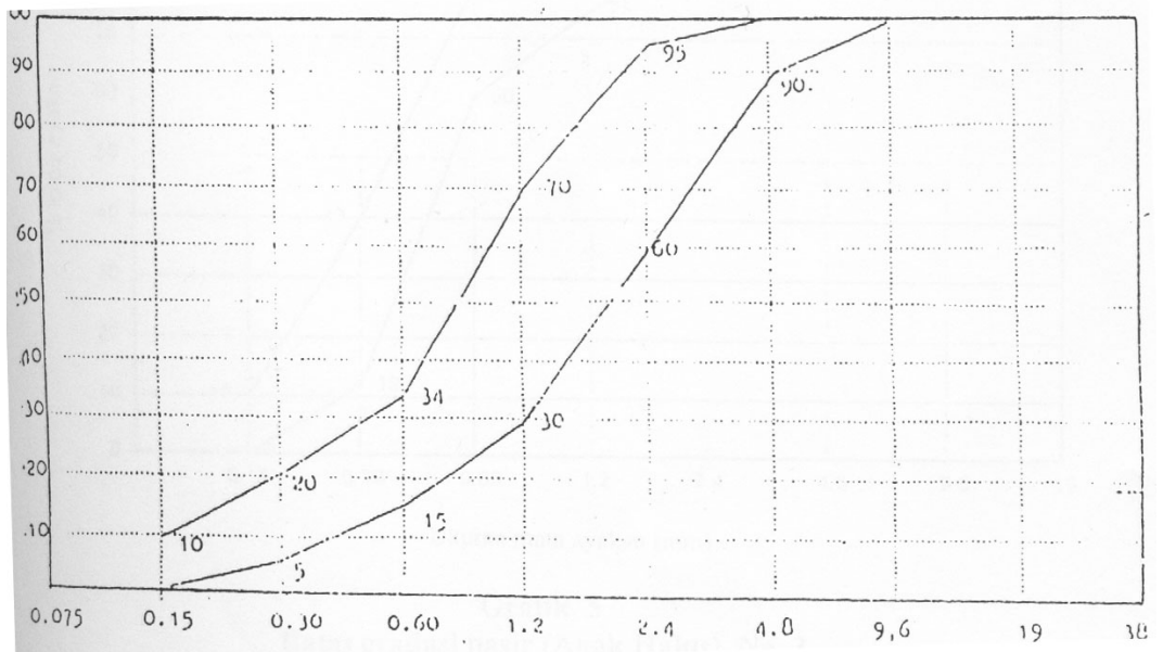
Grafik 3 Batas gradasi pasir (Kasar) No. 1
