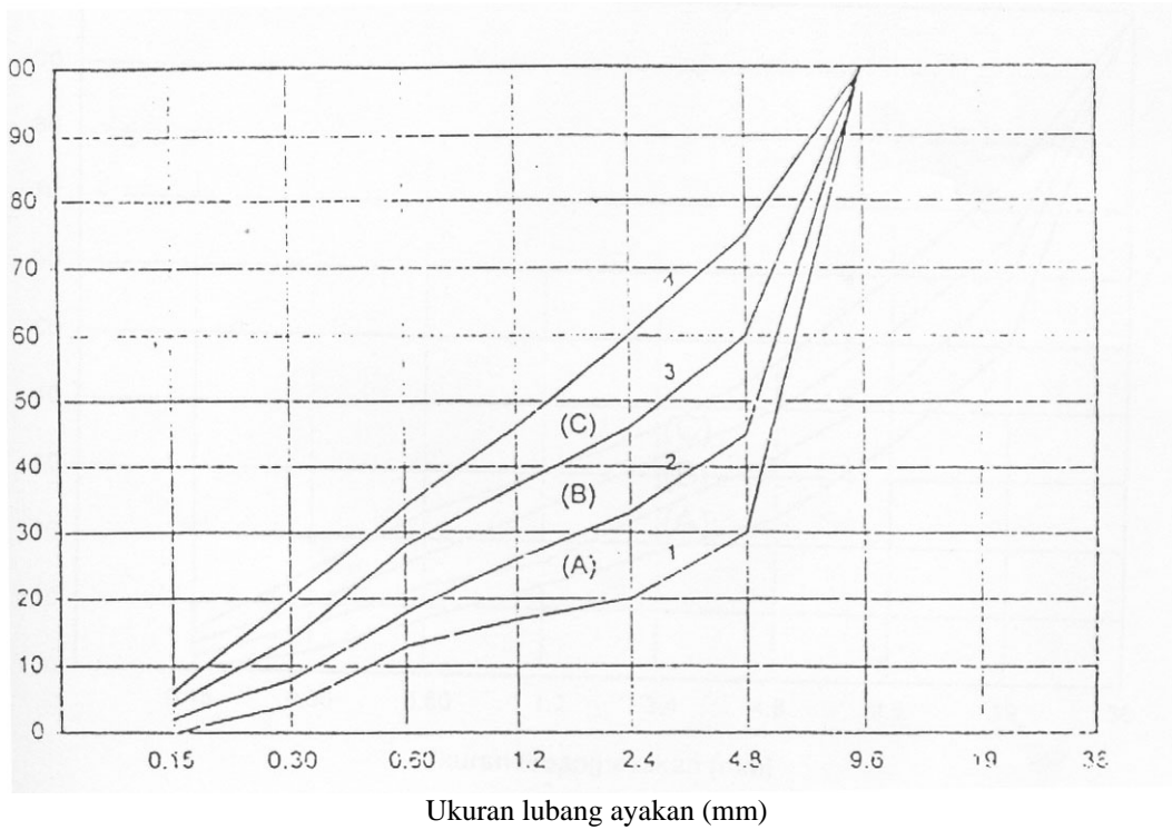
Grafik 10 Batas gradasi agregat gabungan untuk besar butir Maksimum (10mm)
