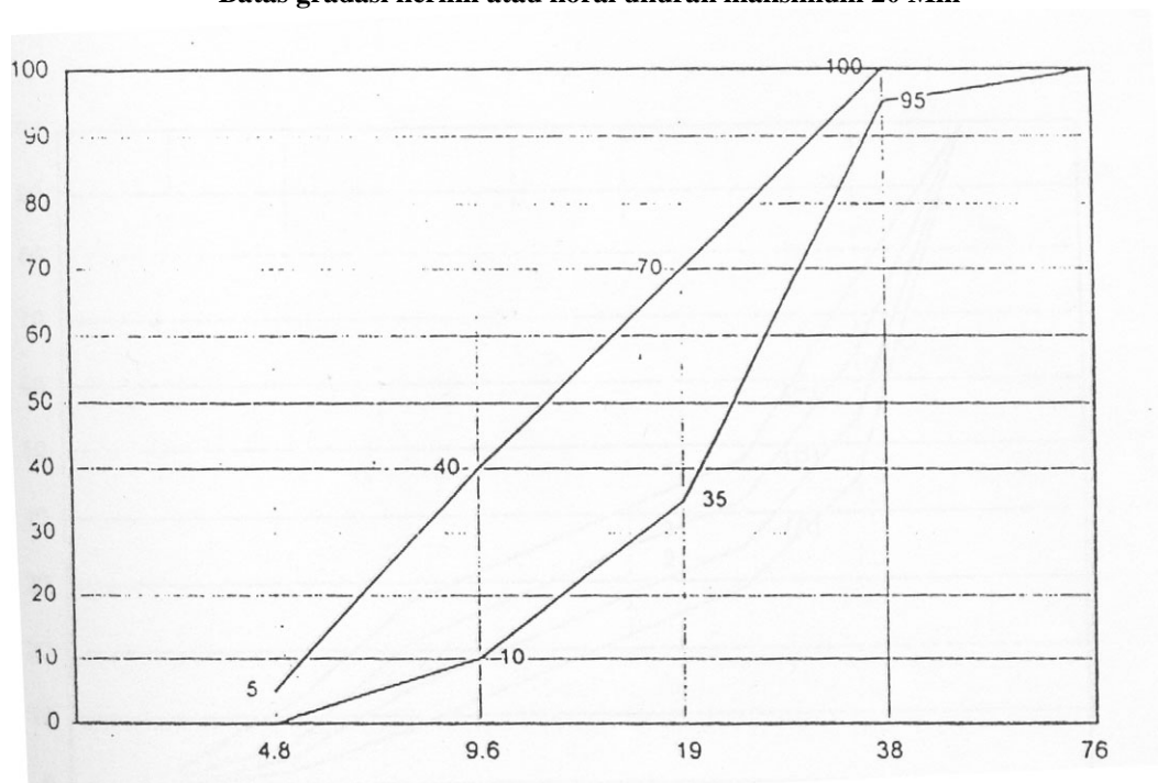
Grafik 8 Batas gradasi kerikil atau koral ukuran maksimum 20 Mm
