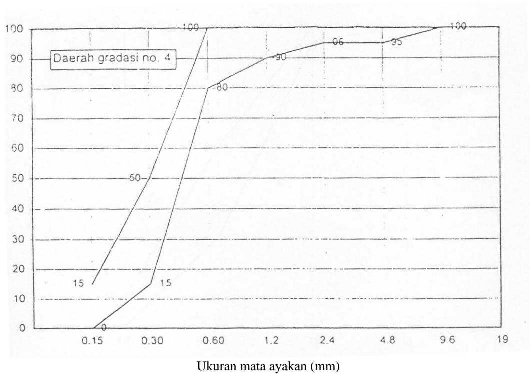
Grafik 6 Batas gradasi pasir dalam daerah No.4
