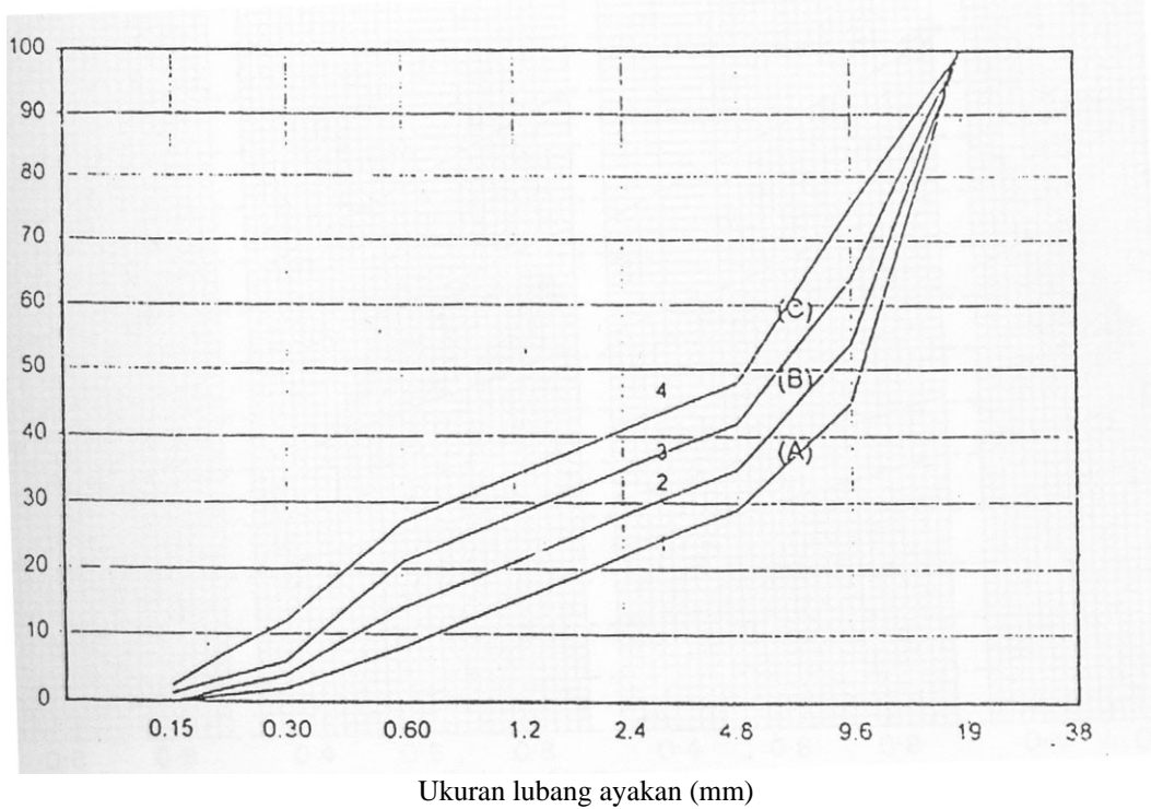
Grafik 11 Batas gradasi agregat untuk besar butir maksimum 20 mm
