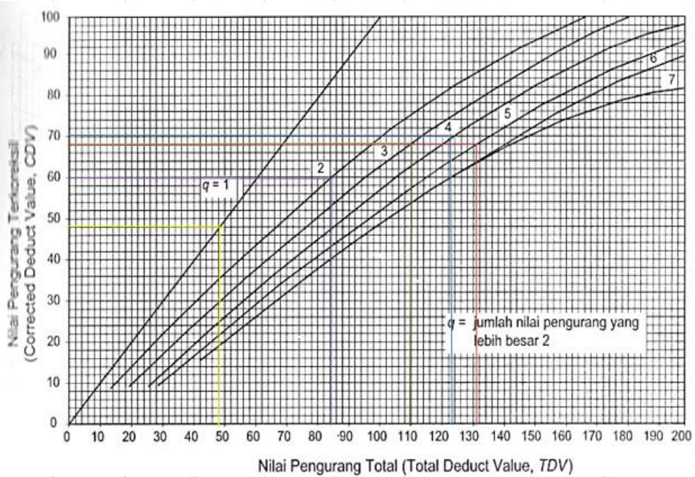
Grafik CDV pada STA 0+500 – 1+000
