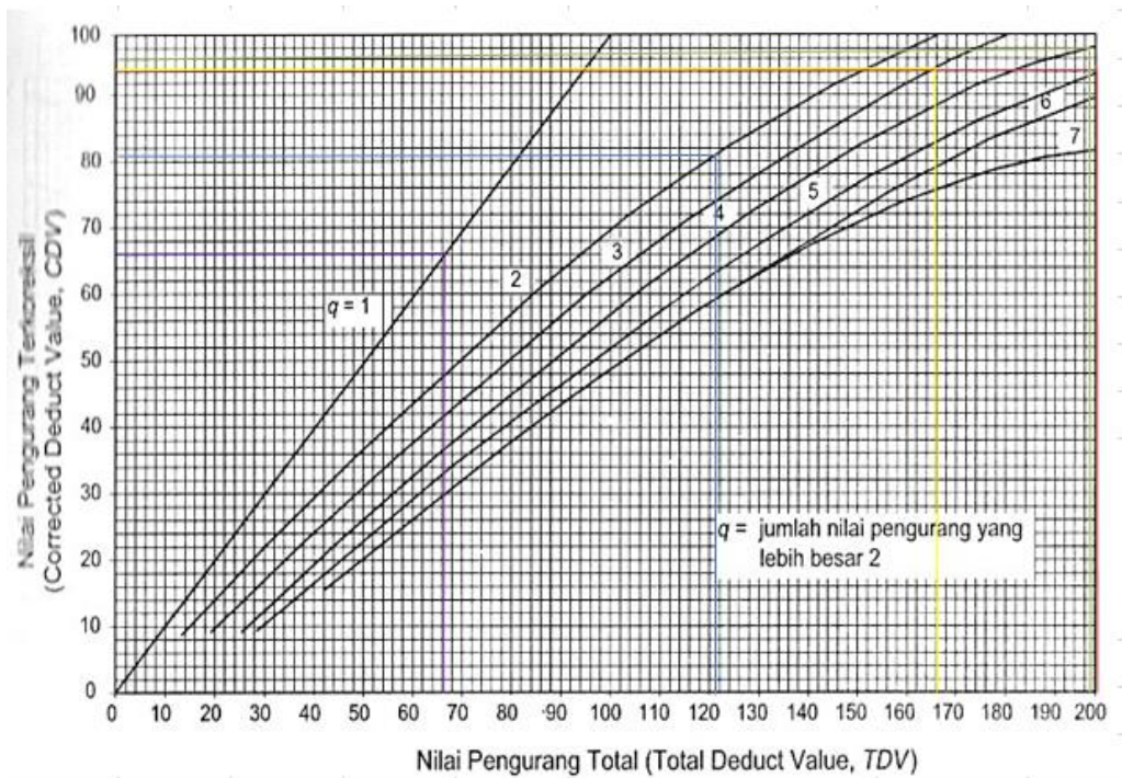
Grafik CDV pada STA 1+500 – 2+000
