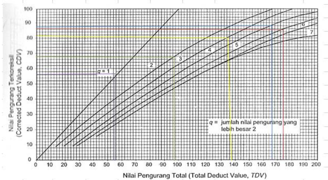
Grafik CDV pada STA 1+000 – 1+500
