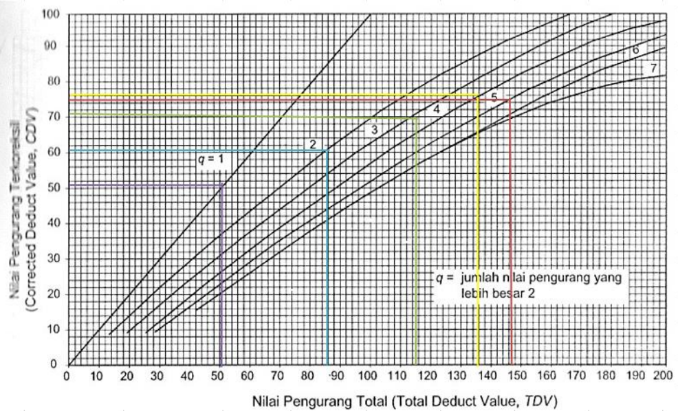
Grafik CDV pada STA 0+000 – 0+500
