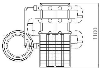
Tampak Atas
