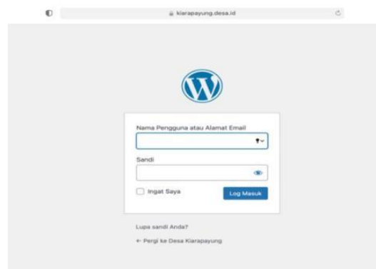
Gambar 50. Halaman Login
